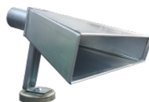
P12000 CAP FIX DE ASPIRARE, DREPTUNGIULAR (400X50MM) Hota de aspirație din oțel zincat pentru colectarea fumurilor sau a prafului în suspensie. Conexiune pentru conducta cu diametrul de 50 mm
